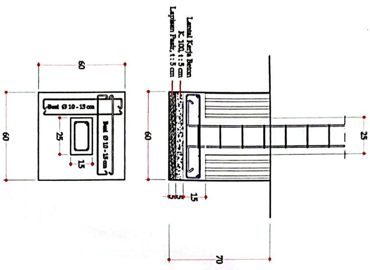
DETAIL PONDASI TAPAK UK. 60x60x15 CM Scale 1 : 20
